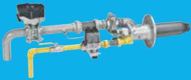
Komplette Beheizungssysteme und Regelstrecken
