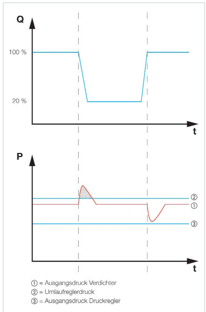
Bild 5: Ansprechverhalten bei plötzlichem Lastwechsel Fig. 5: Reaction behaviour at sudden load change
