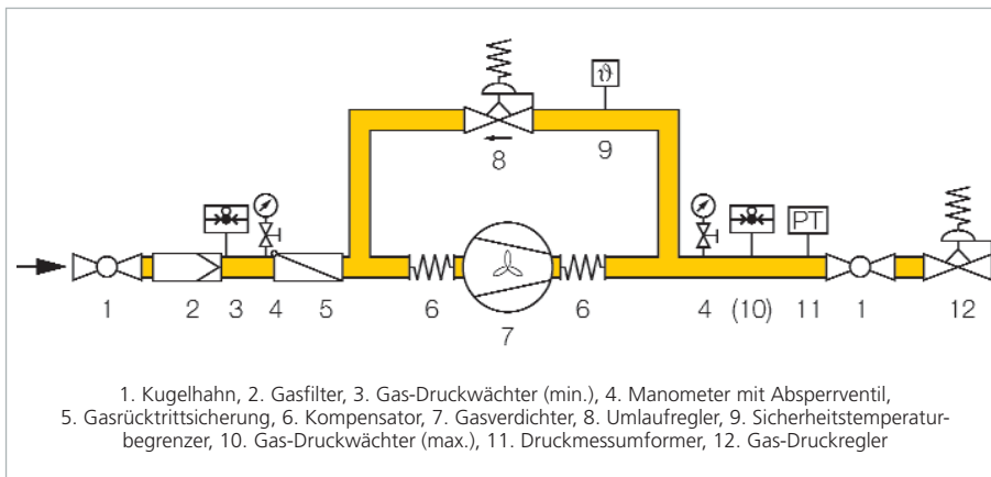
Bild 2: Schematische Darstellung
